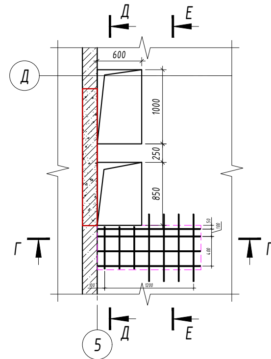
Фрагмент 2 в осях Д/5 на отм. +15,850
