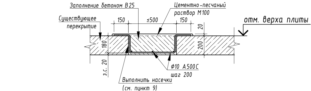
Принципиальная схема восстановления плиты в зоне существующего проёма 500 мм и менее
