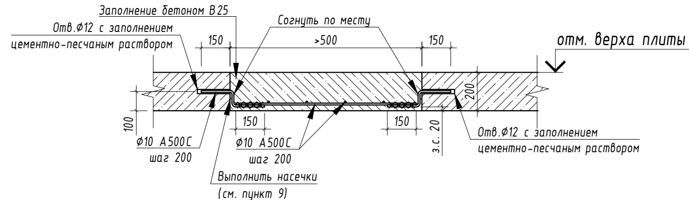
Принципиальная схема восстановления плиты в зоне существующего проёма более 500 мм
