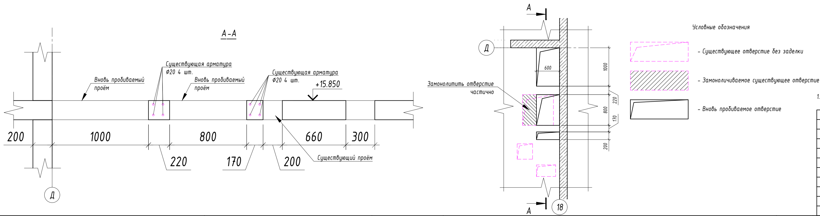
Фрагмент 1 в осях Д/18 на отм. +15,850
